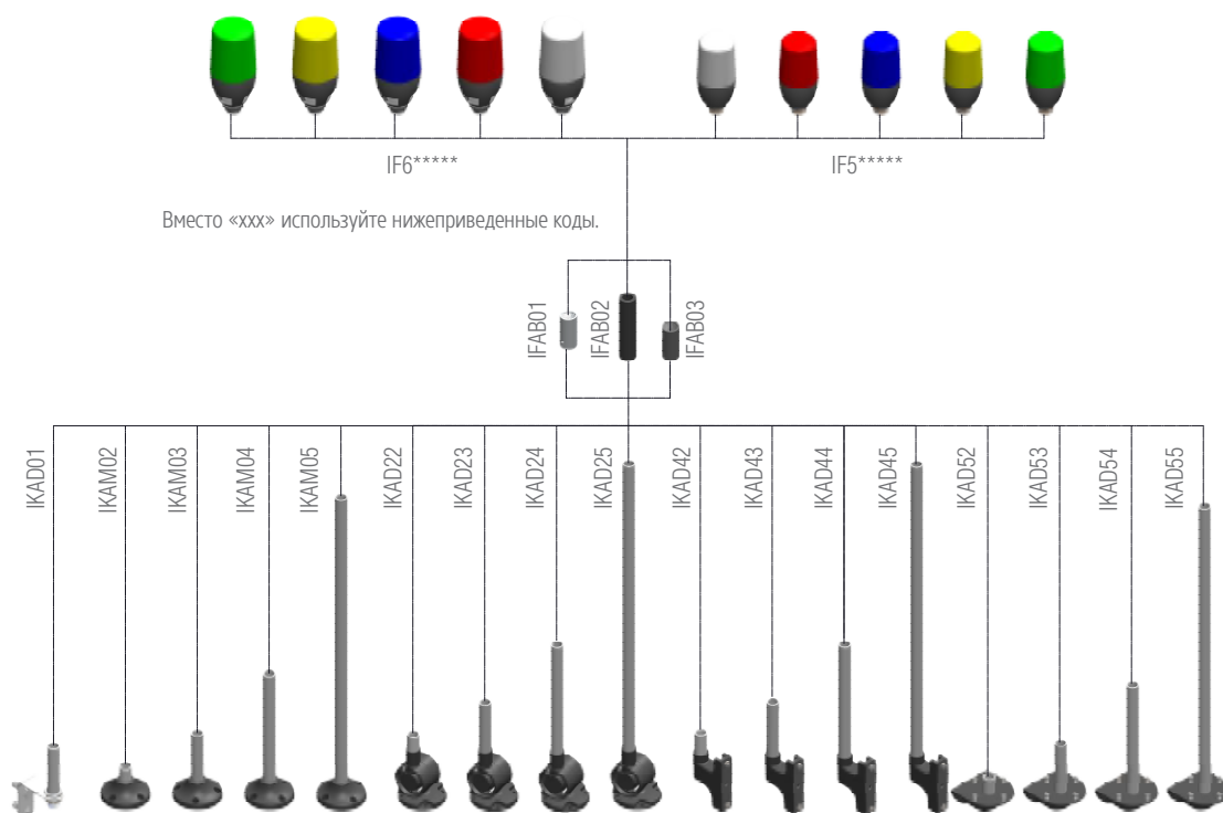
Варианты монтажа серий IF IP65
