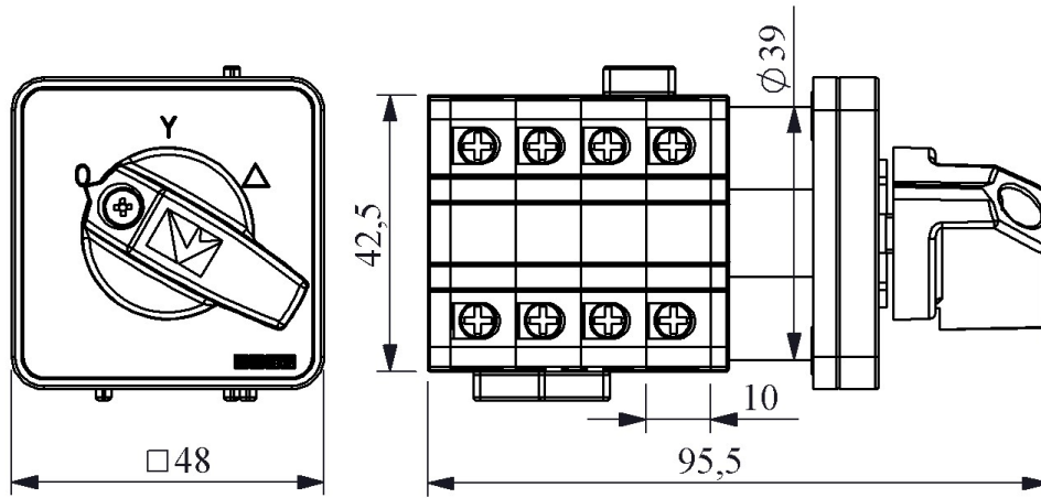
Devre Şeması
